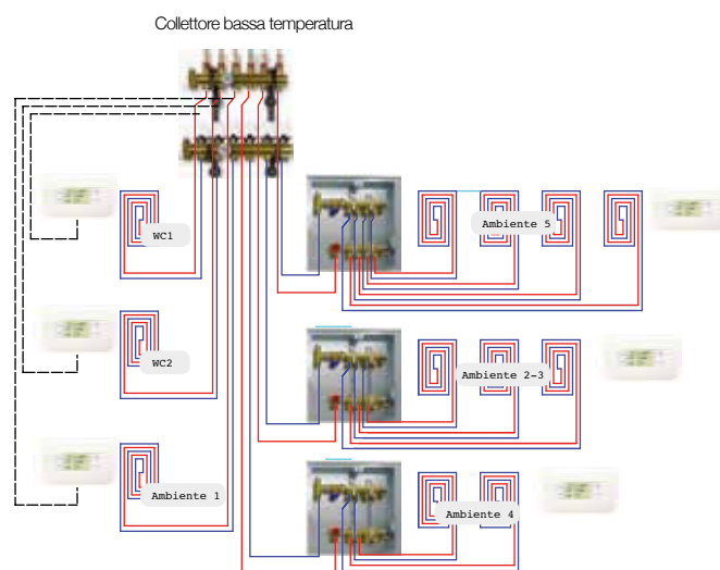
Schema d'impianto
