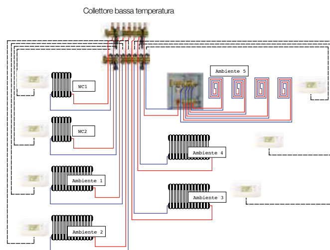
Schema d'impianto
