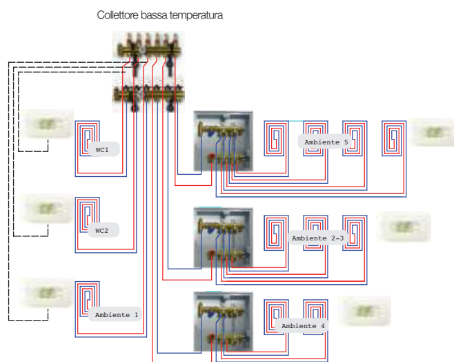
Schema d'impianto
