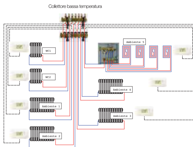
Schema d'impianto
